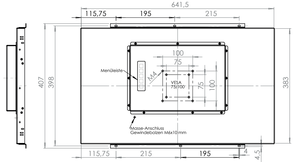
RÜCKANSICHT
